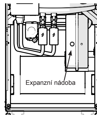
Dolní připojení expanzní nádoby
